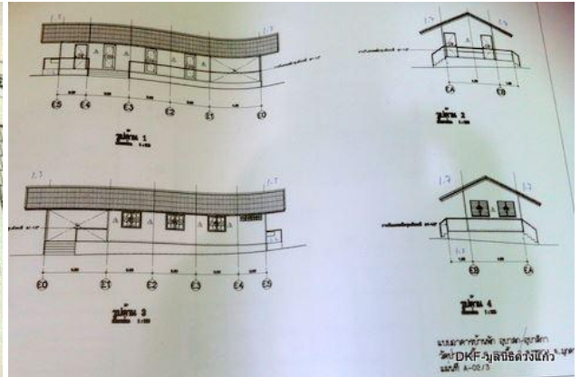
แปลนอาคารพักอุบาสก อุบาสิกา ประมาณ 100 ตรม. มีห้องใต้หลังคาไว้เก็บของด้วย
